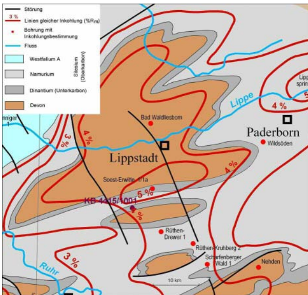
Die Prä-Perm-Oberfläche im Bereich des Lippstädter Gewölbes nach neuesten Bohrungsergebnissen
